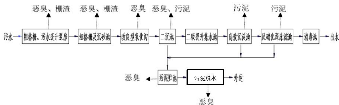
图 2.2-1 兴国县污水处理厂工艺流程图
